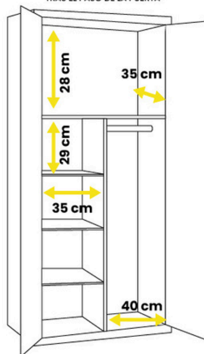
DIMENSIONES ÚTILES TRAS EL PASO DE LA PUERTA
