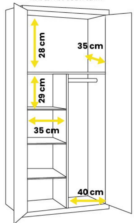
DIMENSIONES ÚTILES TRAS EL PASO DE LA PUERTA
