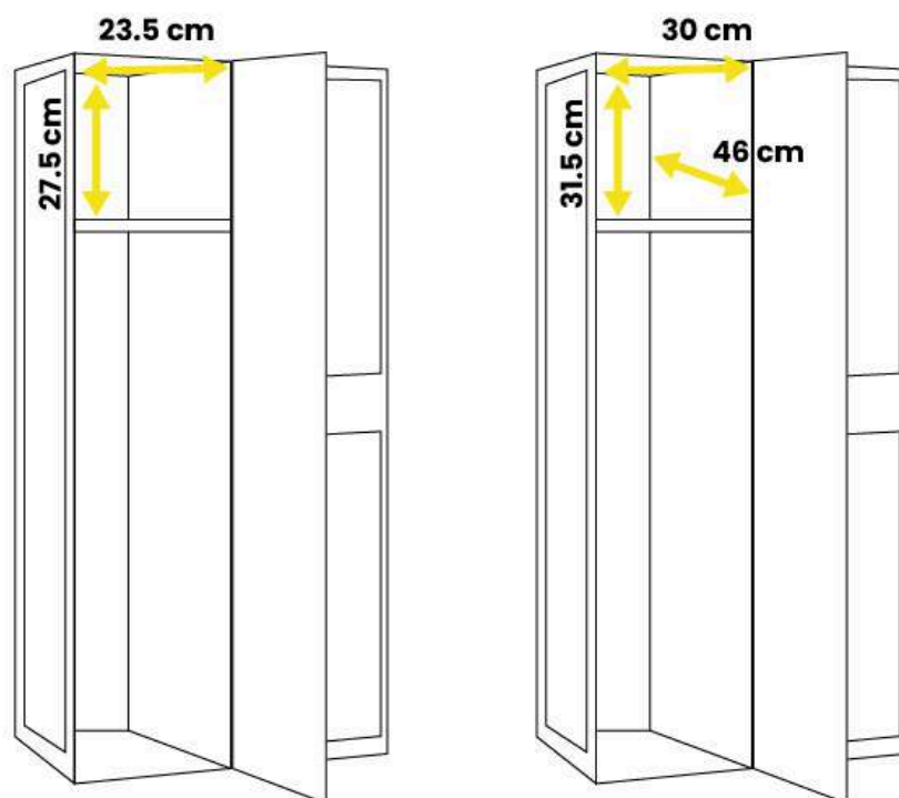
DIMENSIONES DEL ESPACIO DE PASO DE LA PUERTA
